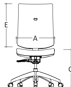
VTM3 A : 19 1/2" C : 17 3/4 - 22 3/4" E : 23"
