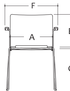
AGPS-D2 A : 18" C : 28" E : 15" F : 22 1/2"
